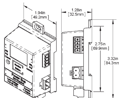
Current Output Module
