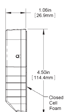
BAPI-Stat 2 Enclosure
