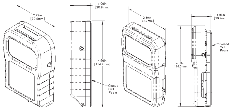
BAPI-Stat 2 Enclosure
