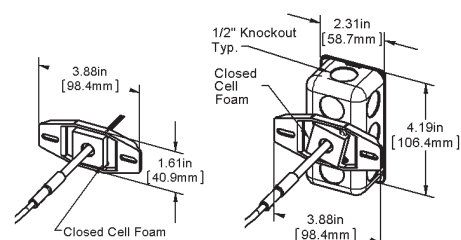
No Box (NB)
