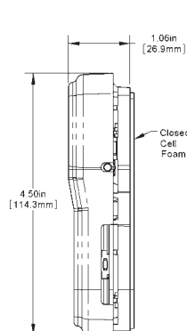
BAPI-Stat 4 Enclosure
